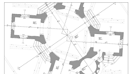
Grundriss - Haus der Laune, Laxenburg | AT
