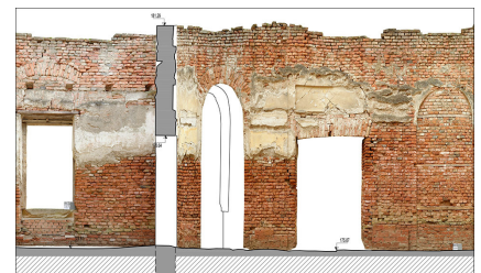
Schnitt mit Abwicklung - Haus der Laune, Laxenburg | AT
